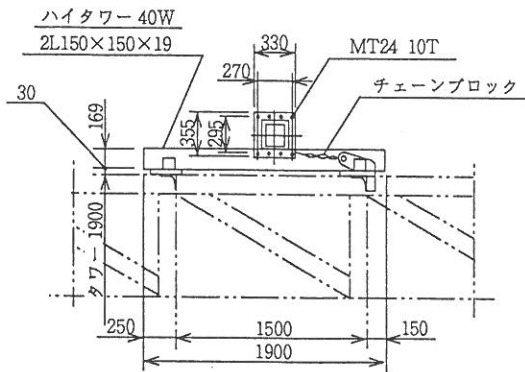
A 矢視
