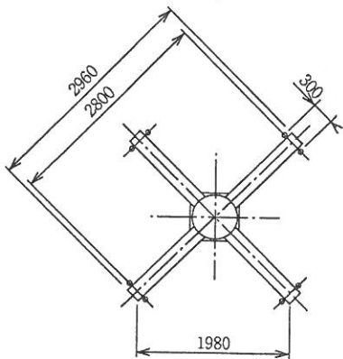
● ベース平面図
