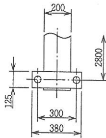
● ベースアンカー詳細図
