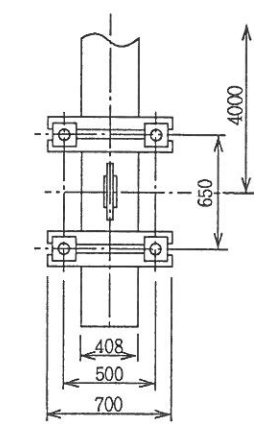
● ベースアンカー詳細図
